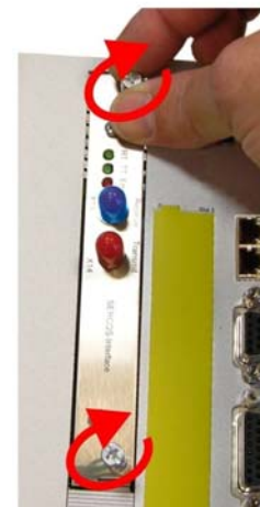
9 – Затяните винты
